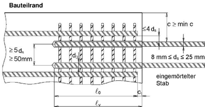
Bild 7: Allgemeine Konstruktionsregeln für eingemörtelte Bewehrungsstäbe
