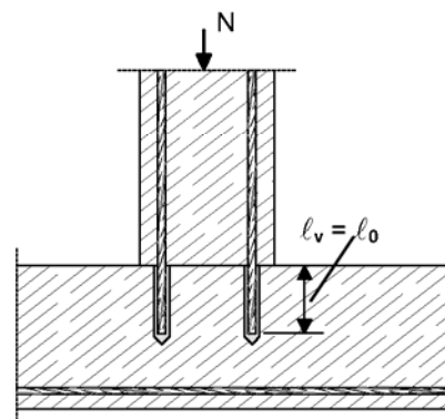
Bild 4: Bewehrungsanschluss überwiegend auf Druck beanspruchter Bauteile.
