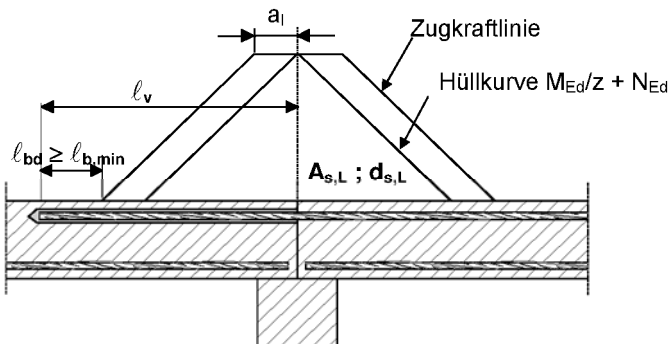
Bild 5: Verankerung von Bewehrung zur Deckung der Zugkraftlinie
